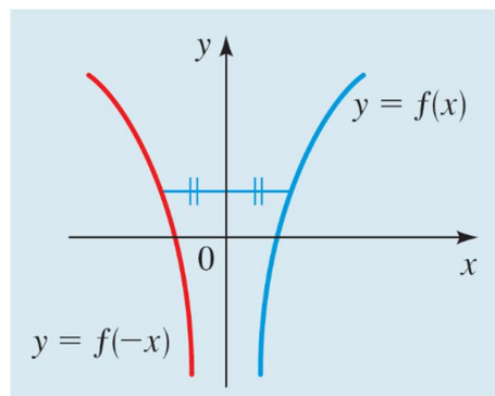
تغيير إشارة متغير الدالة يعكس الرسم حول y -axis
